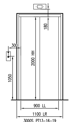
3000S_PT13-16-19 ДЛЯ ВЫЗЫВНОГО ПОСТА ЭТАЖ 1, А Масштаб 1:25
