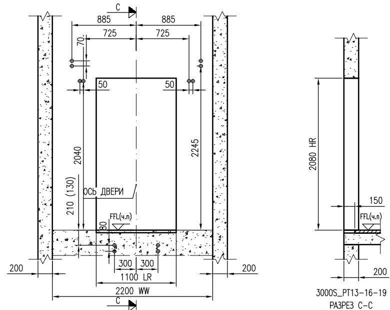
3000S_PT13-16-19 ВИД ИЗ ШАХТЫ, СТРОИТЕЛЬНЫЙ ПРОЕМ Масштаб 1:25
