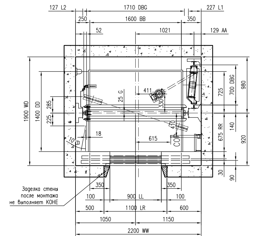
ПЛАН ШАХТЫ И КАБИНЫ: 3000S_PT13-16-19 Масштаб 1:20
