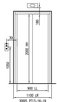
3000S_PT13-16-19 ДЛЯ ВЫЗЫВНОГО ПОСТА ЭТАЖ 2 - 17, А Масштаб 1:25
