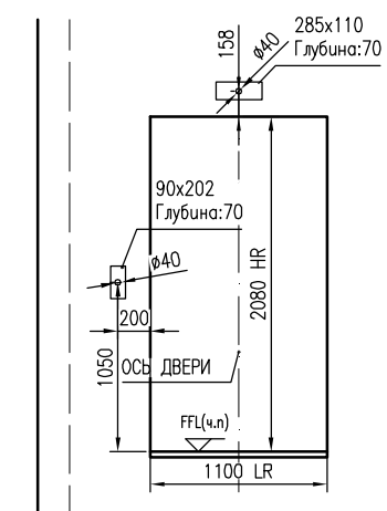
3000S_PT13-16-19 ВИД НА ДВЕРЬ, ЭТАЖ 2 - 17, А СТРОИТЕЛЬНЫЙ ПРОЕМ Масштаб 1:25
