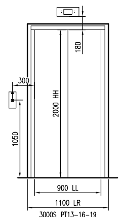
3000S_PT13-16-19 ДЛЯ ВЫЗЫВНОГО ПОСТА ЭТАЖ 18, А Масштаб 1:25
