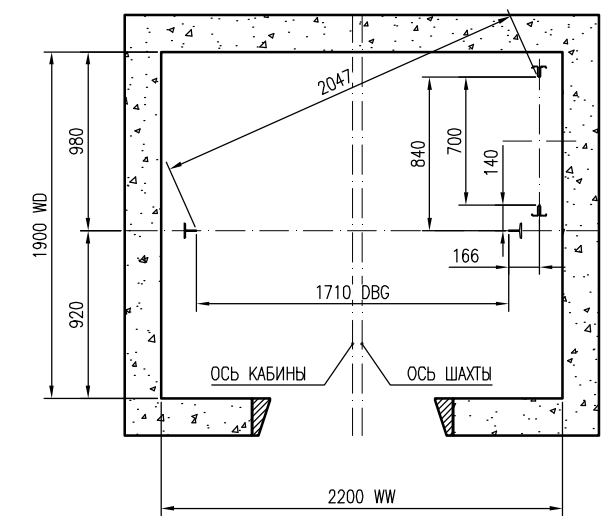
НАПРАВЛЯЮЩИЕ: 3000S_PT13-16-19 Масштаб 1:20
