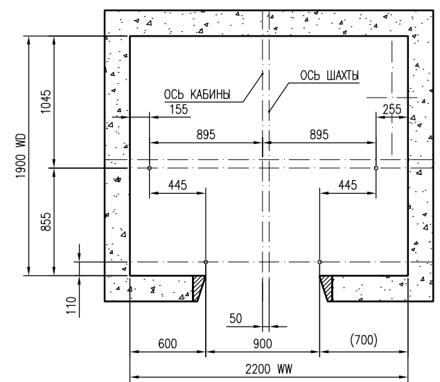
ПРОВЕСКА ШАХТЫ: 3000S_PT13-16-19 Масштаб 1:20
